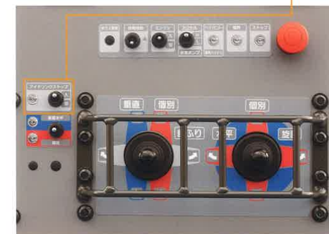
上部操作部
