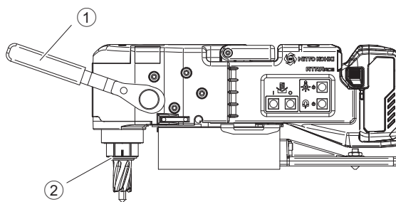
① 送りハンドル ② アーバ
