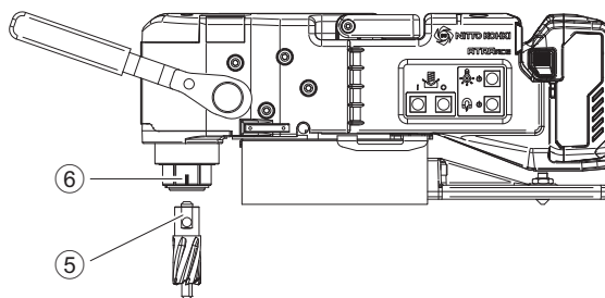
⑤ くぼみ部 ⑥ スリーブ
