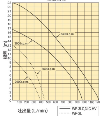
性能曲線
