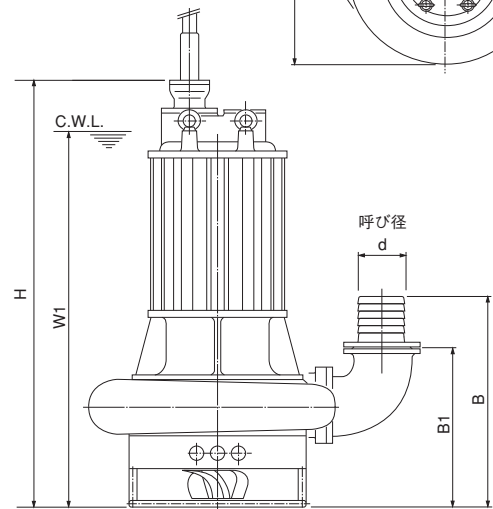
寸法表
