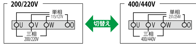
カムスイッチ (三相⇄単相切替)
