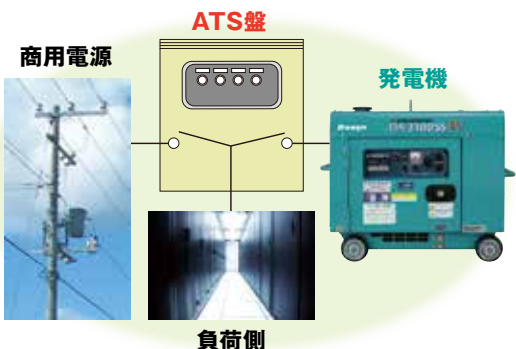
自発停型発電機※1 電源切替盤(ATS盤)※2
